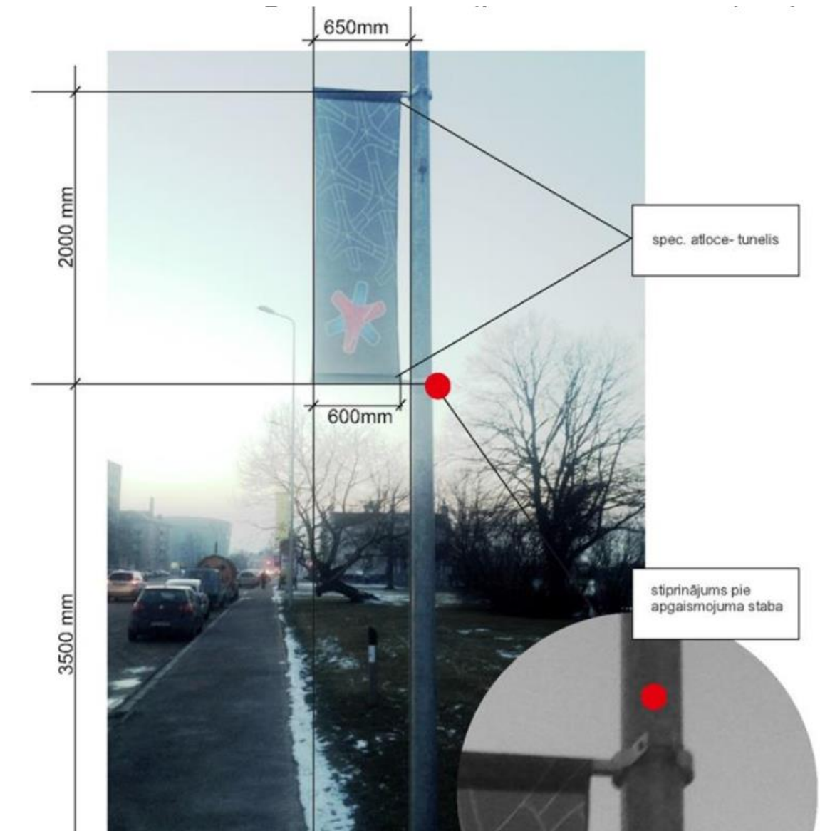
Lipu mōdud
