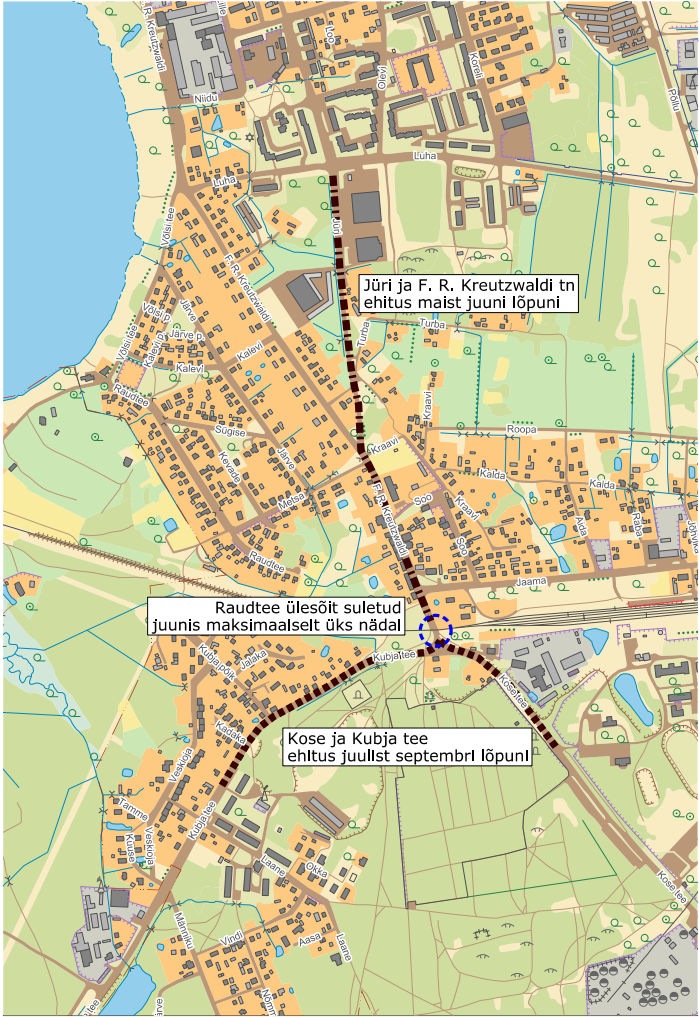
Tööde esialgne ajagraafik ja liikluskkeem.
