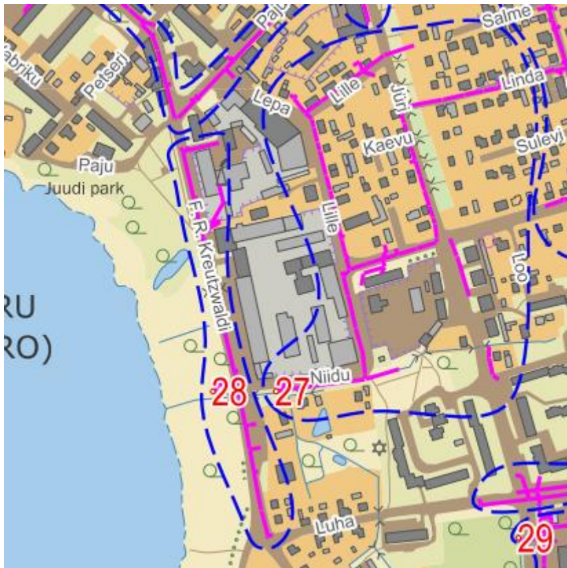
Lisa 2.3 Skeem: sademeveesüsteemid 27 ja 28
